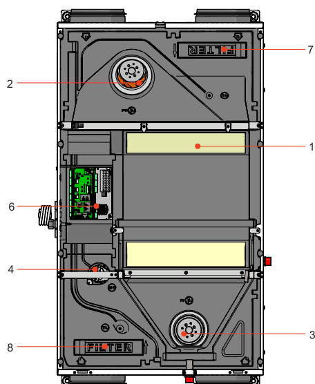
Abbildung 4.4.1. Smarty 2 XP Aufbau
