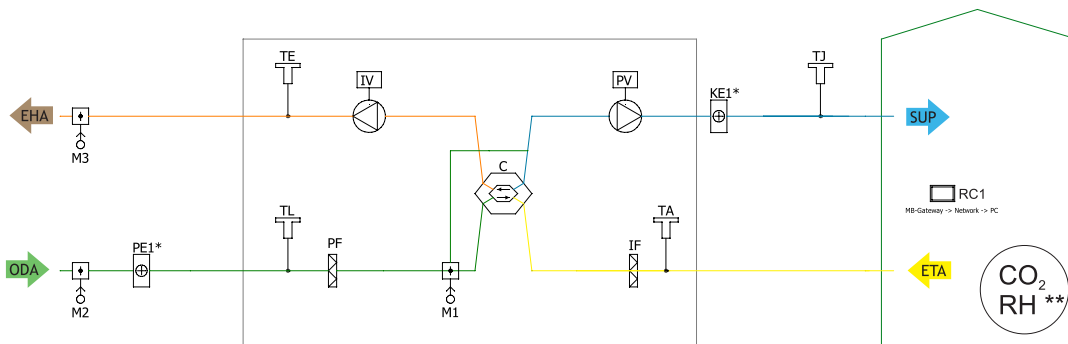
Abbildung 6.6.2. Smarty XP 1.2 *Es kann nur ein Heizgerät (Vorheizregister oder Heizregister) angeschlossen werden; **Sehen Sie für mehr Details in die Anleitung
